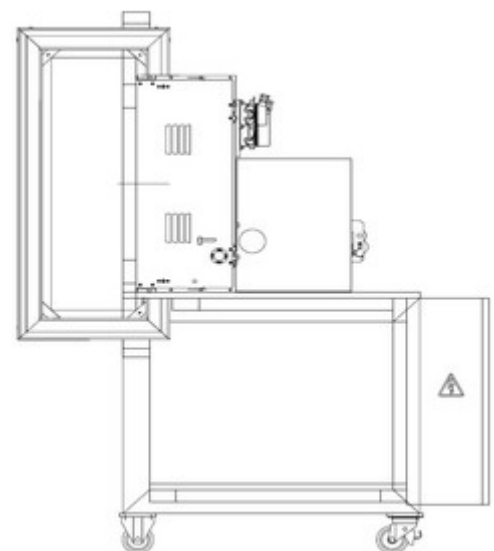
Teststand für OMS Umreifungsköpfe
